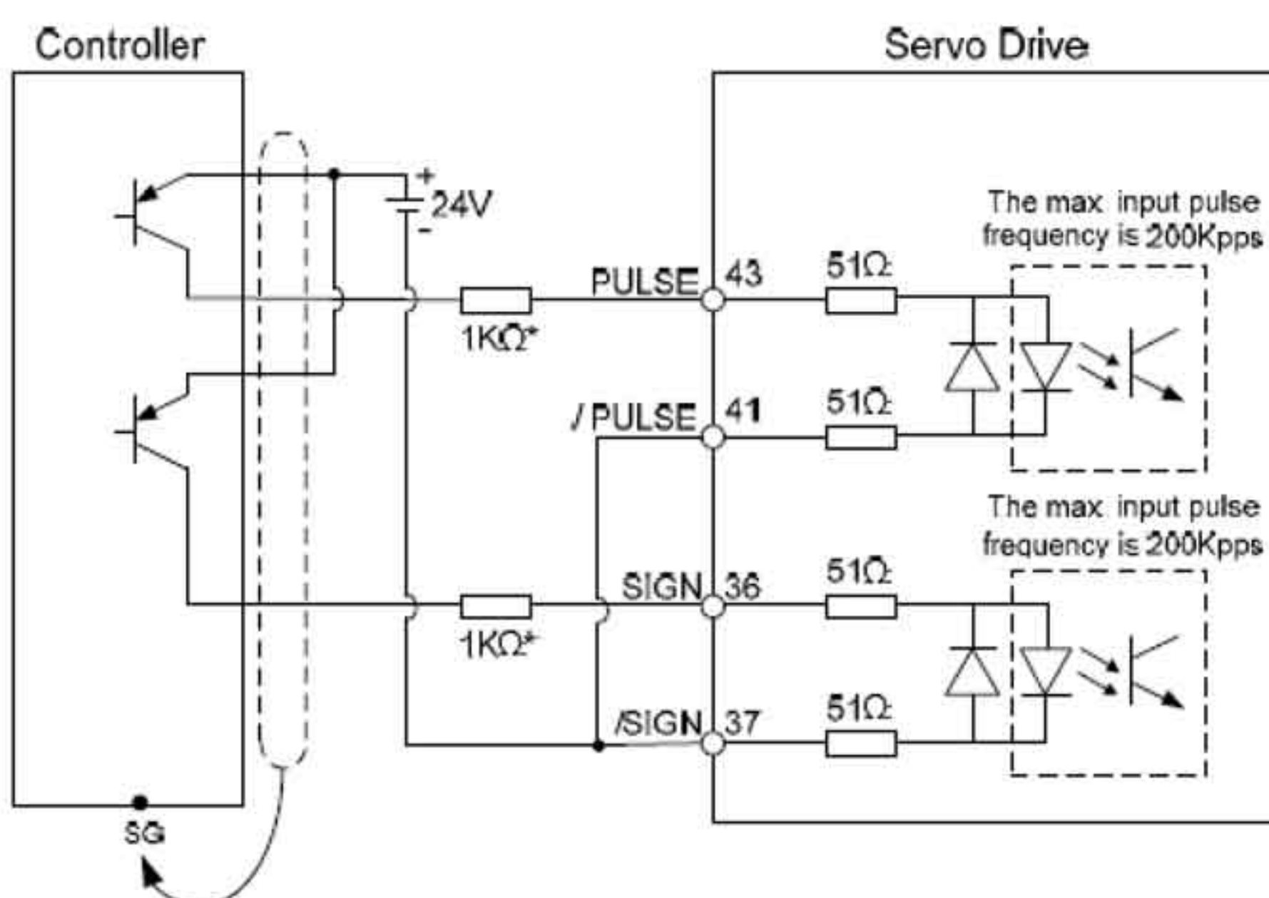
С3-4: Импульсы с открытого коллектора PNP с использованием внешнего источника питания
