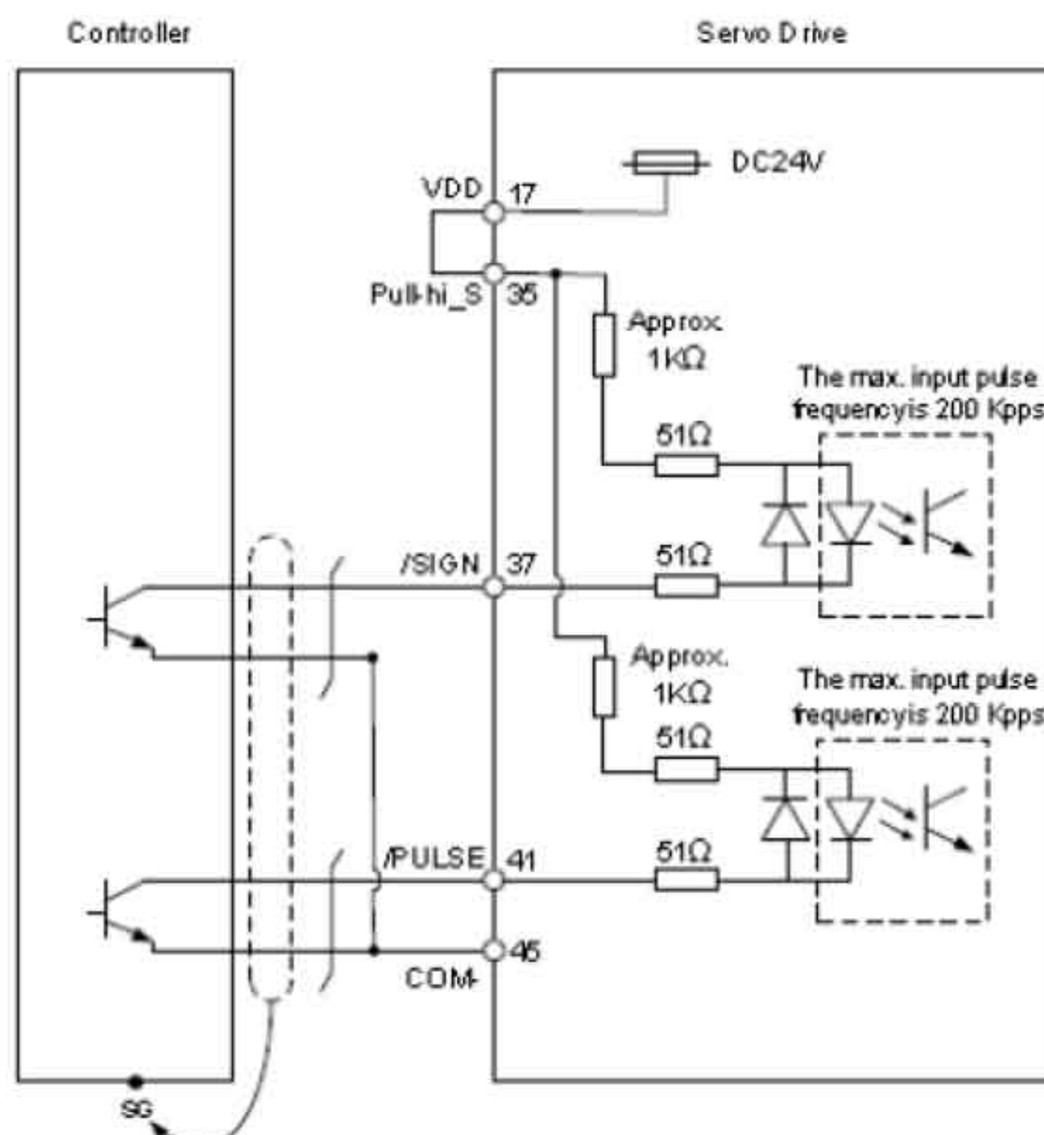
С3-1: Импульсы с открытого коллектора NPN с использованием внутреннего источника питания
