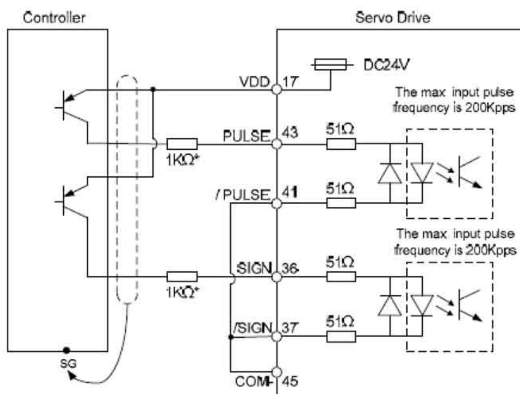
С3-2: Импульсы с открытого коллектора PNP с использованием внутреннего источника питания
