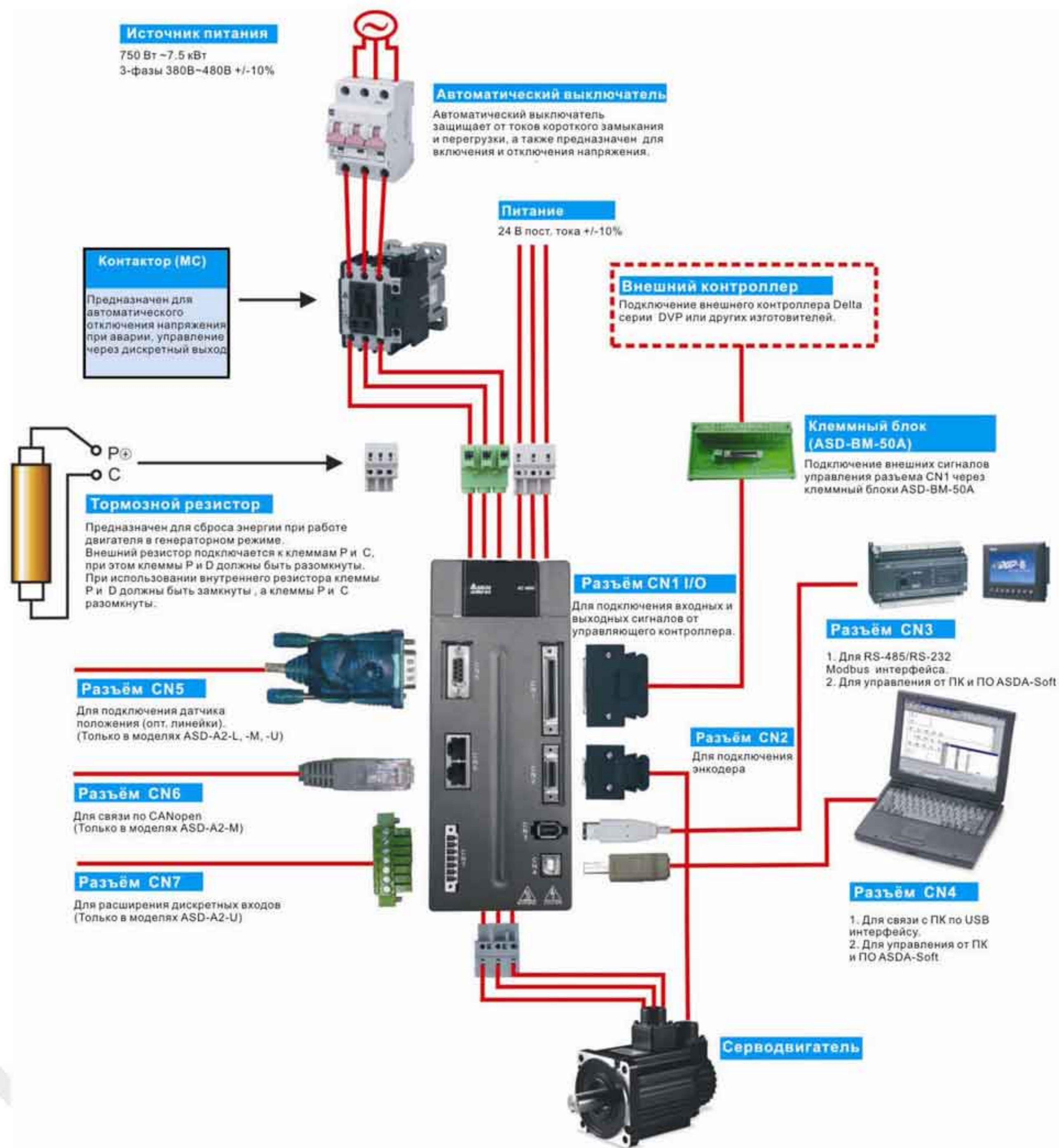
Рисунок 3.4. Конфигурация
