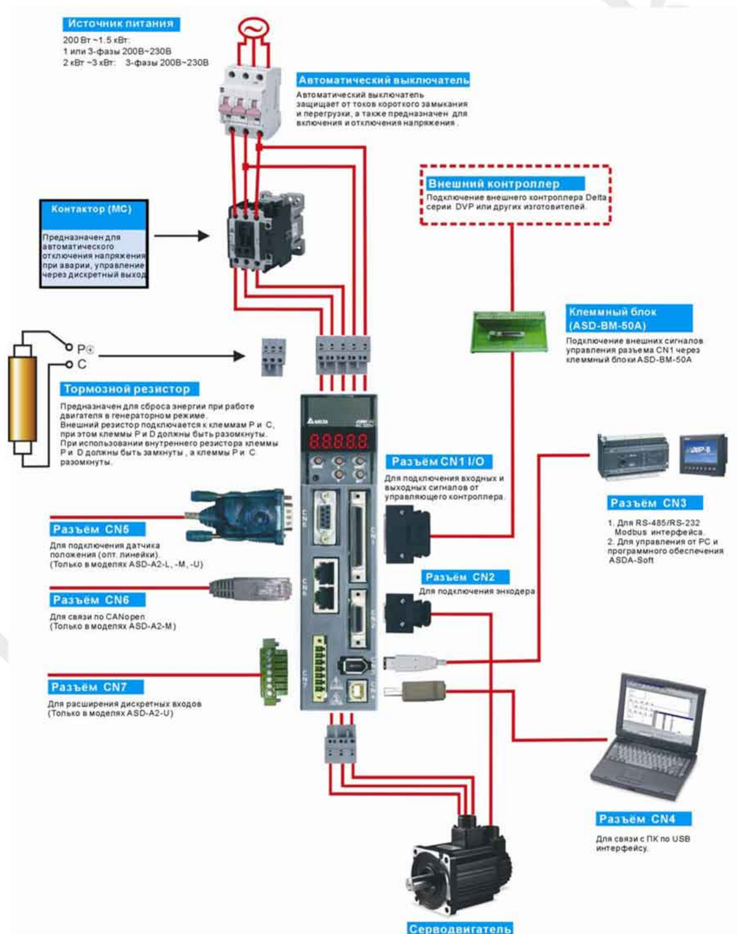
Рисунок 3.1. Конфигурация
