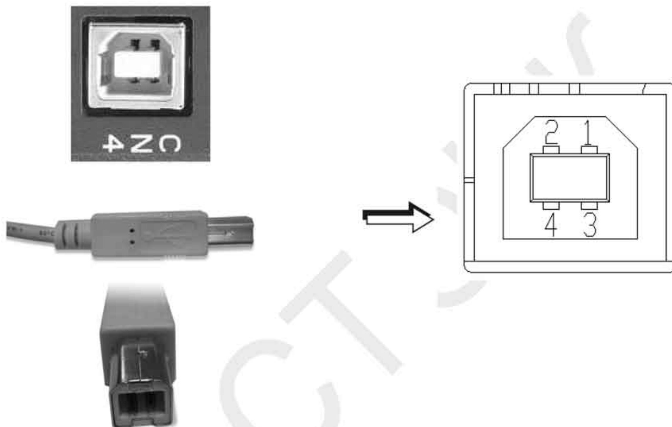
Рис. 3.15. Разъём CN4
