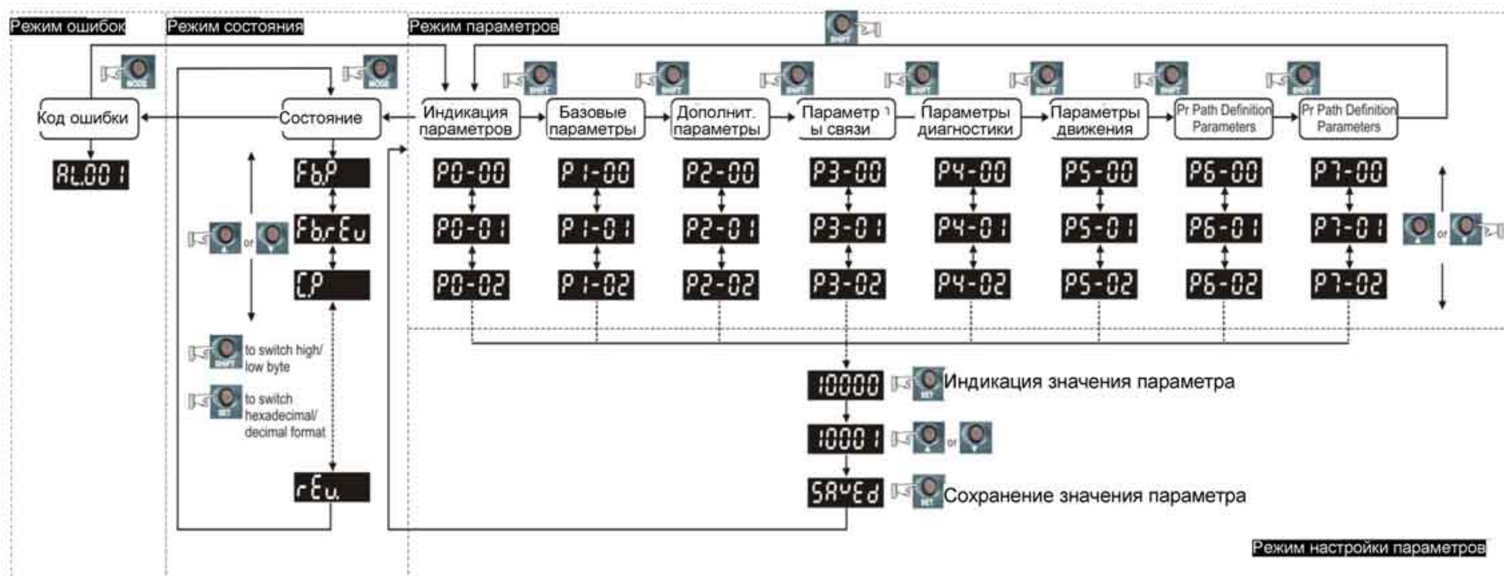
Рис. 4.2 Использование клавиш
