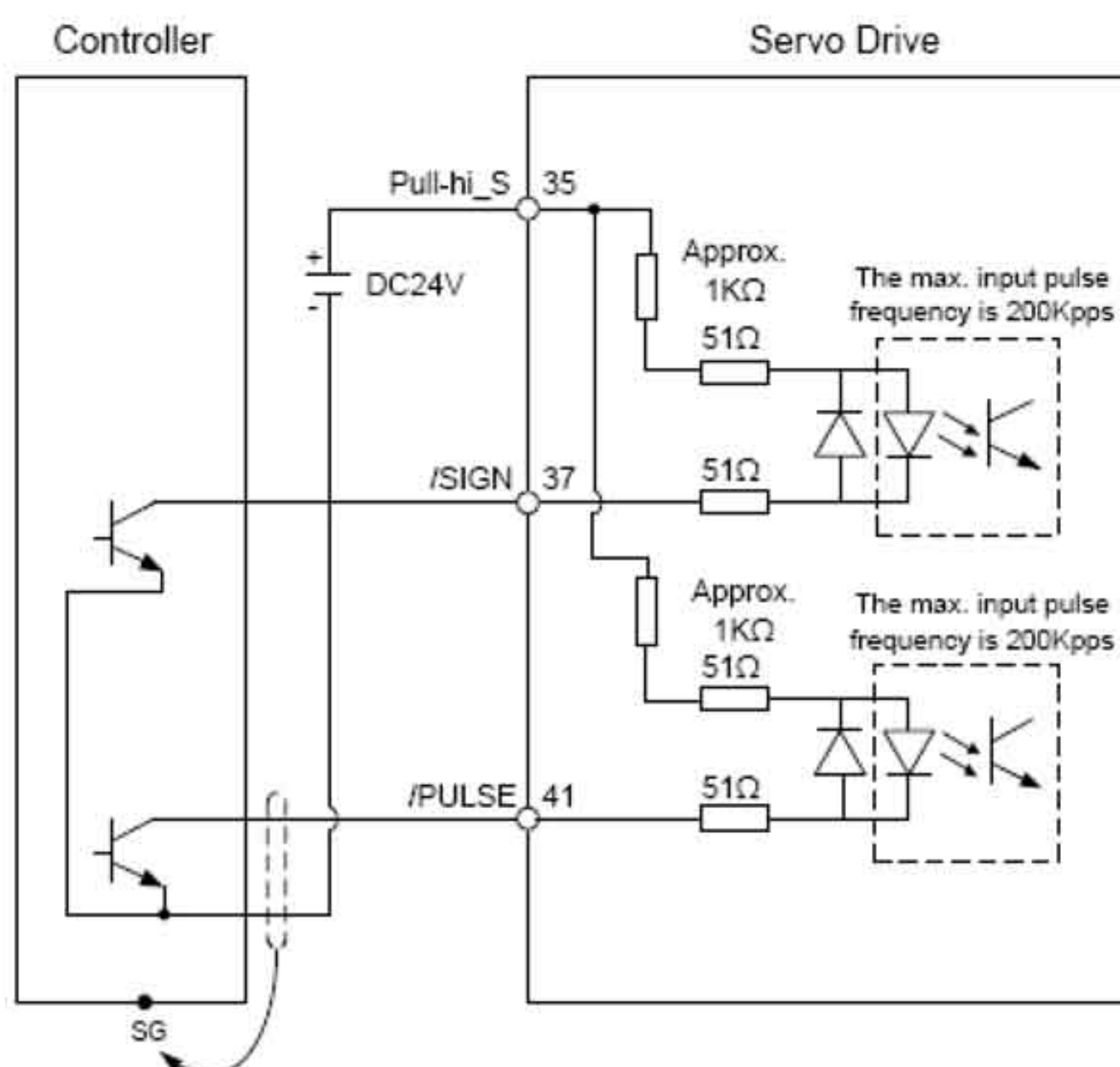
C3-3: Импульсы с открытого коллектора NPN с использованием внешнего источника питания
