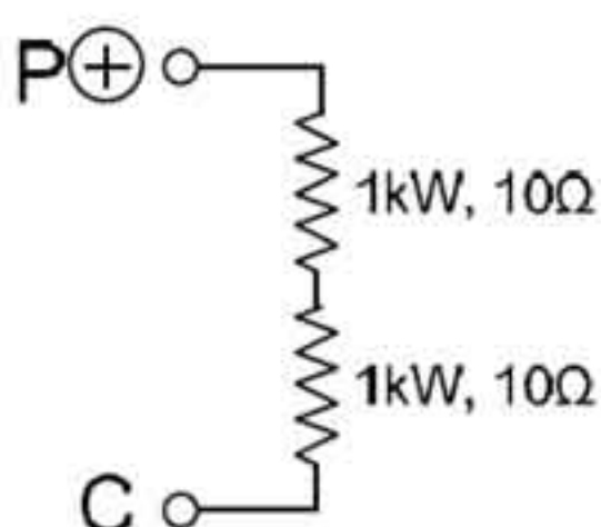
Последовательное соединение
