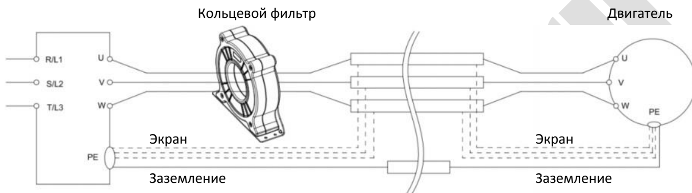
Рисунок А: Установка кольцевого фильтра с одним витком на экранированный кабель
