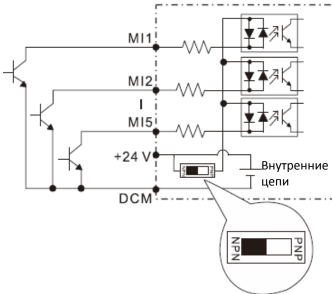
(3) Режим NPN (SINK)
