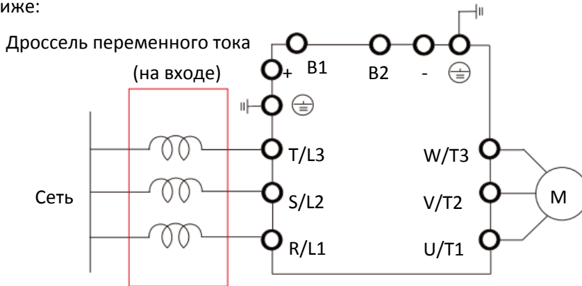
Подключение сетевого дросселя
