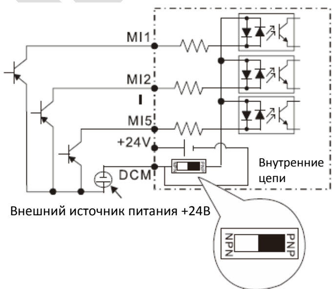
(4) Режим PNP (SOURCE)
